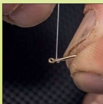
5. Obtočte ramínko háčku 10 až 12 krát
