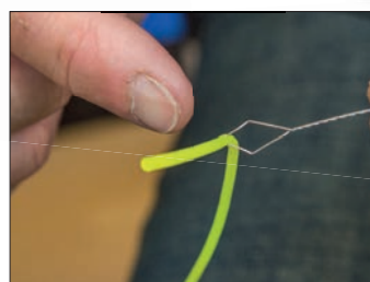
19. Amortizér provlečte očkem struny
