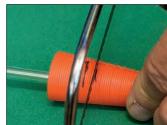
12. Opatrně ořízněte kónus. Kónus otáčejte, abyste nerozřízli průhlednou trubičku
