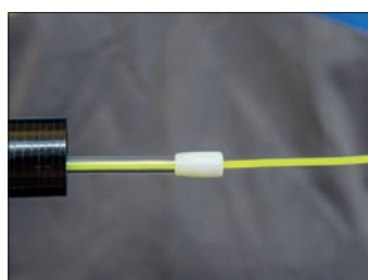
22. Kónus vtačte do děličky a protáhněte amortizér
