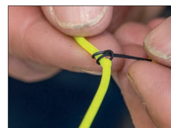
24. Těsně pod uzlem připevněte Dacron konektor provlečením skrz smyčku a pevně utáhněte
