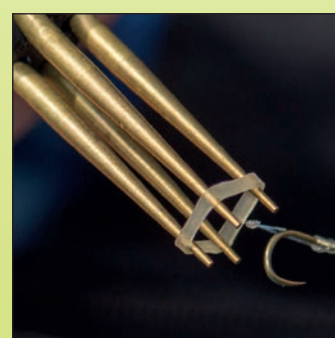
8. 6 mm peletu vložte do gumičky pomocí Pellet Bander
