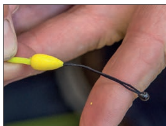
26. Zatlačte gumový korálek konektoru přes uzel
