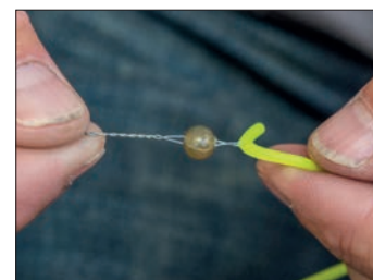
28. Navlečte korálek na strunu
